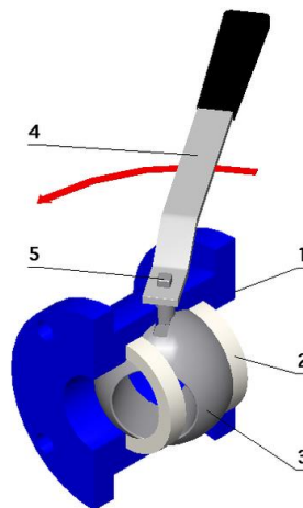
Figure 7.3: 1.) Body 2.) Head 3.) Ball 4.) Lever handle 5.) Stem 59
